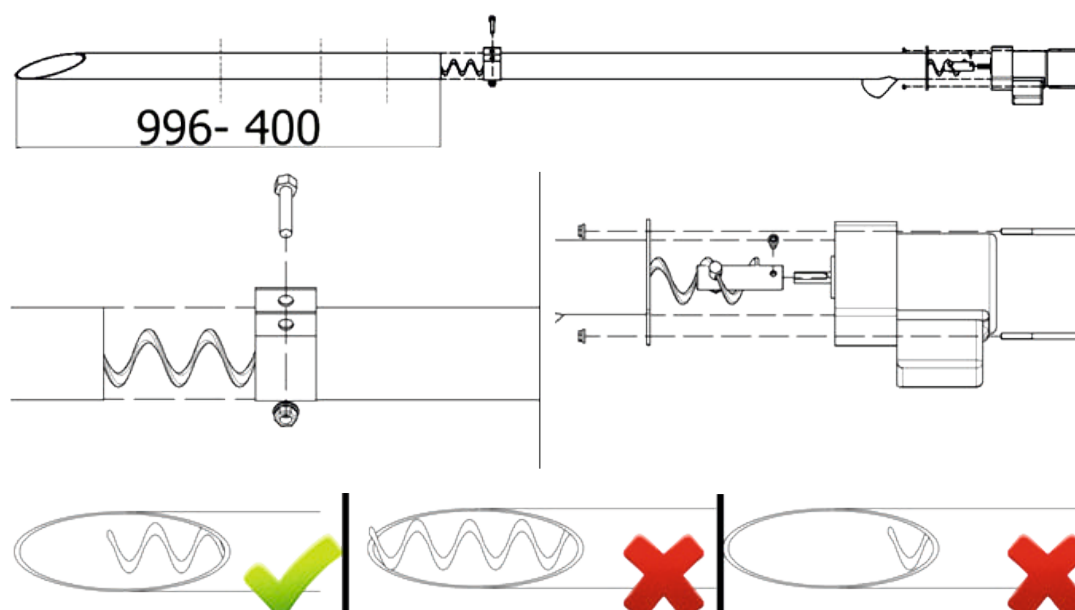
Рисунок 7. Схема установки винтового подающего устройства в штучере бункера
