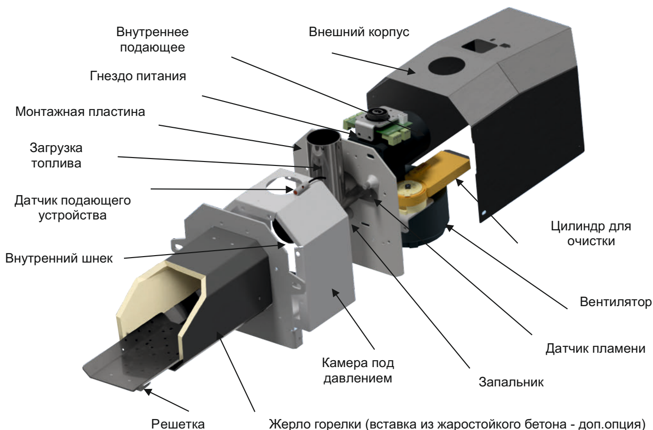
Рисунок 6. Состав Горелок Lavo Eco 25-100
