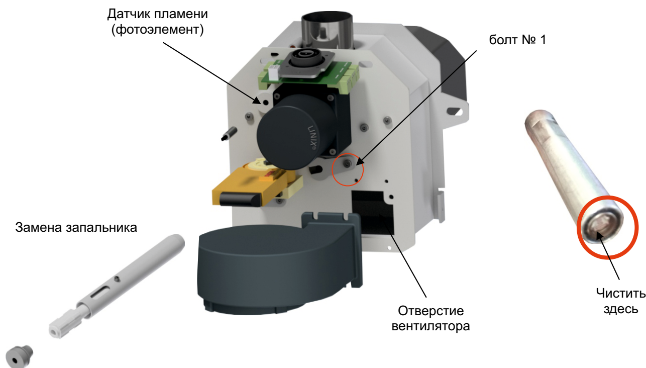
Рисунок 5. Схема демонтируемых узлов для очистки и ревизии
