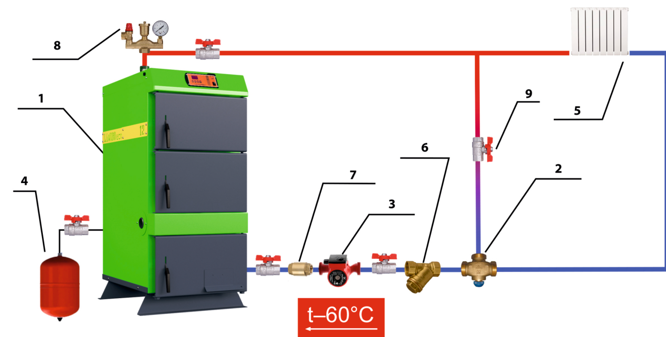
Рисунок 2. Типовая схема обвязки котла Lavoro Eсо с баком-аккумулятором
