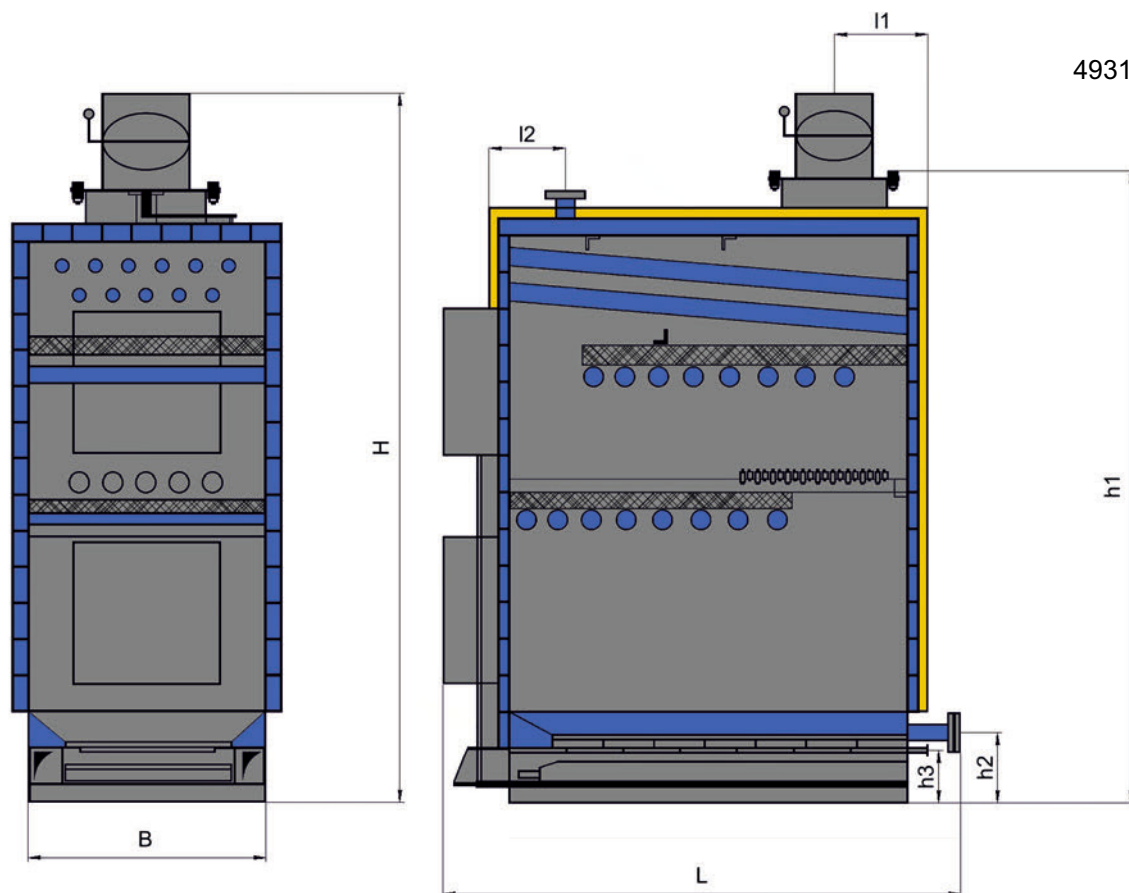
Рисунок 1 - Габаритные и присоединительные размеры Котлов моделей Р 150 - 500 базовой комплектации.
