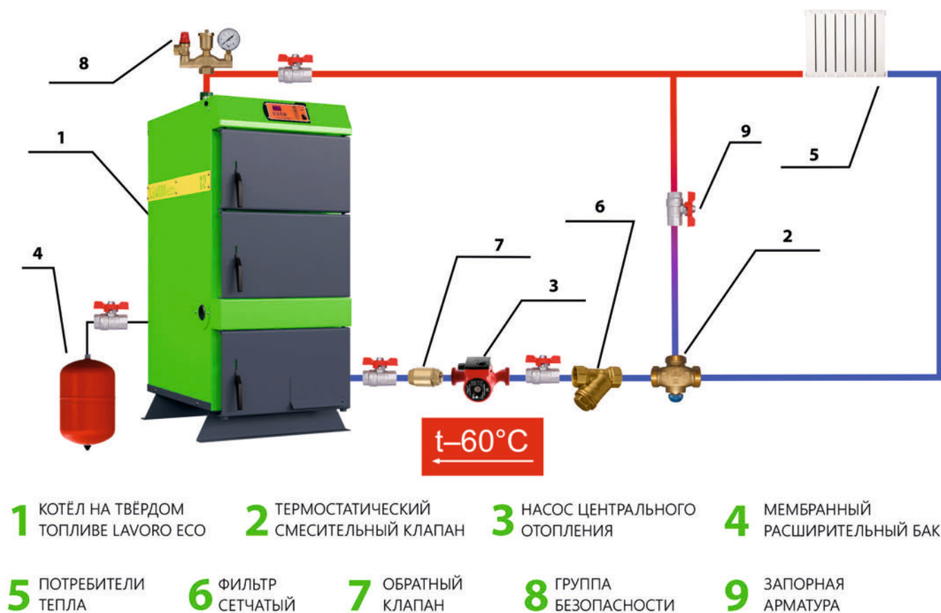
Рисунок 5. Типовая схема обвязки котла с 3-х ходовым клапаном
