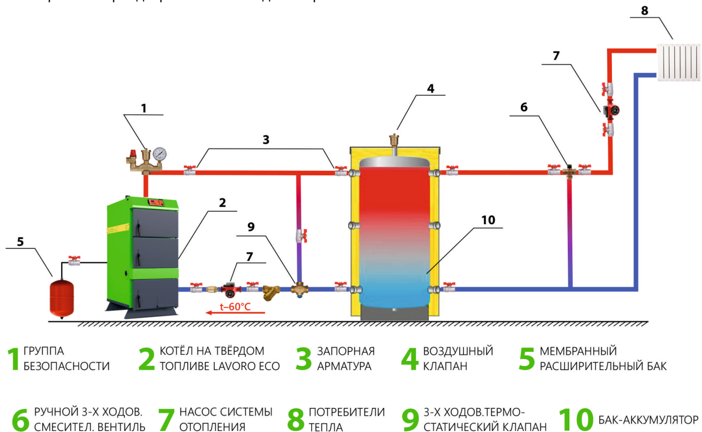
Рисунок 3. Типовая схема обвязки котла Lavoro Eco с баком-аккумулятором
