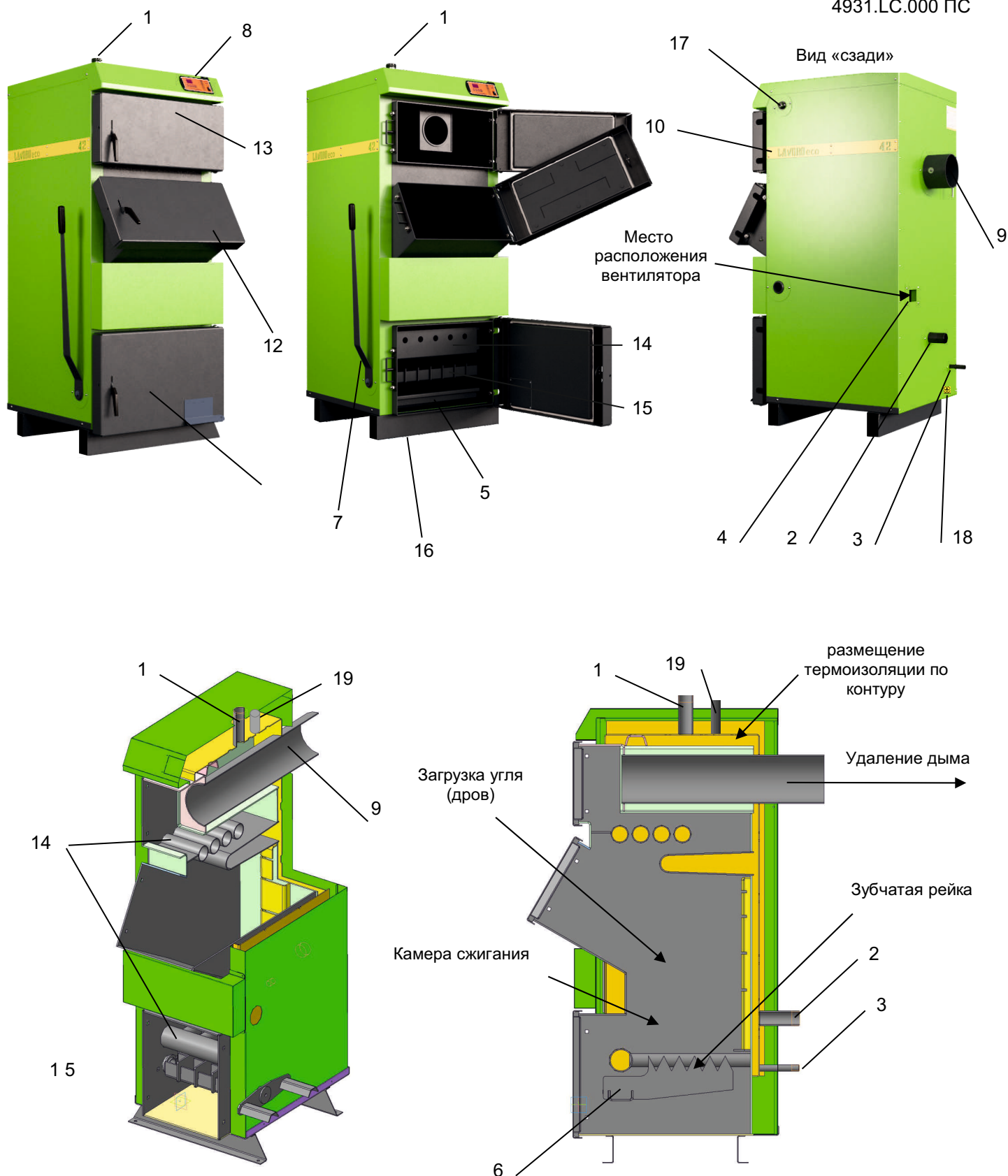
Рисунок 2. Состав и устройство Котлов моделей LC12-52
