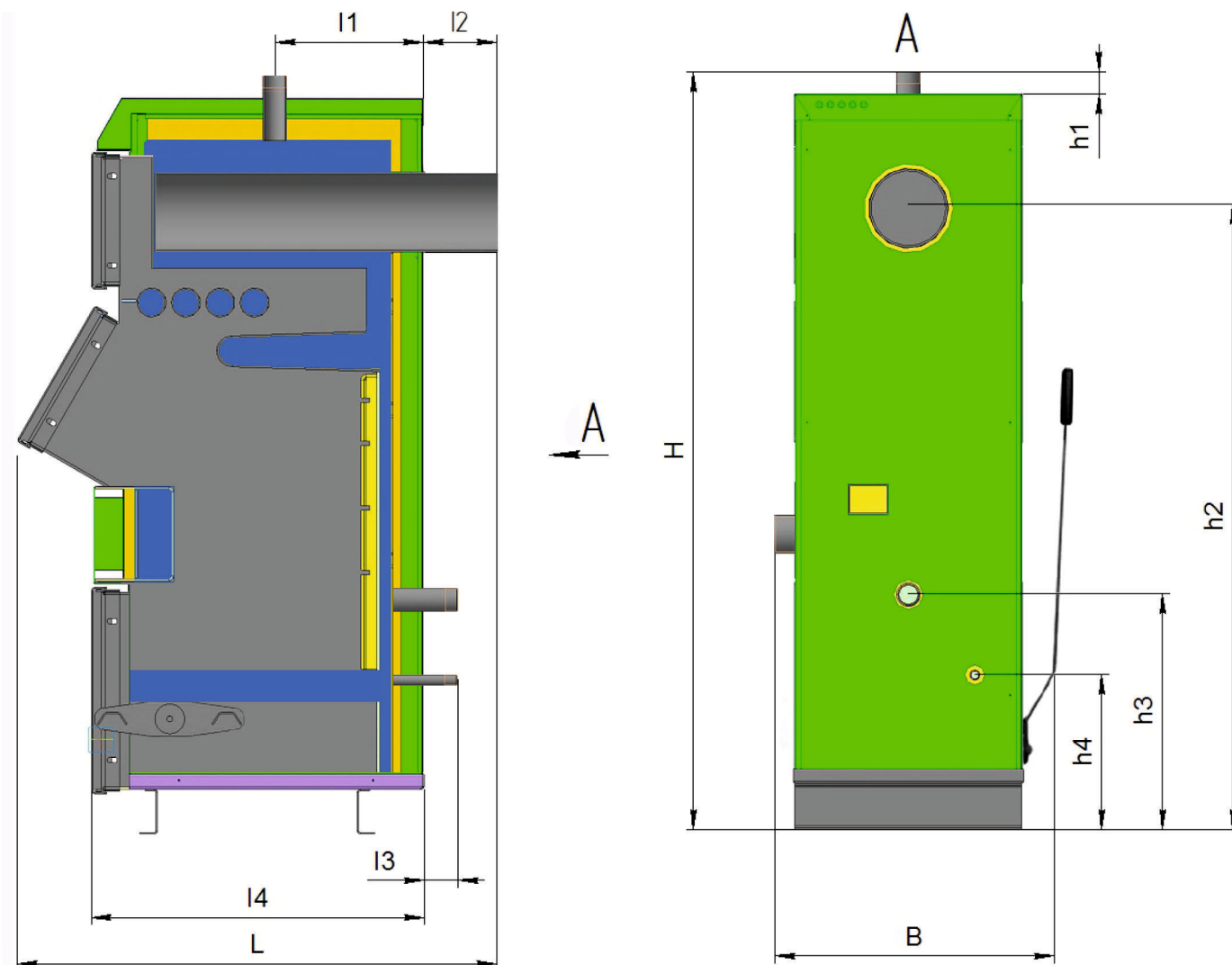
Рисунок 1. Габаритные и присоединительные размеры Котлов моделей LC 12-52
