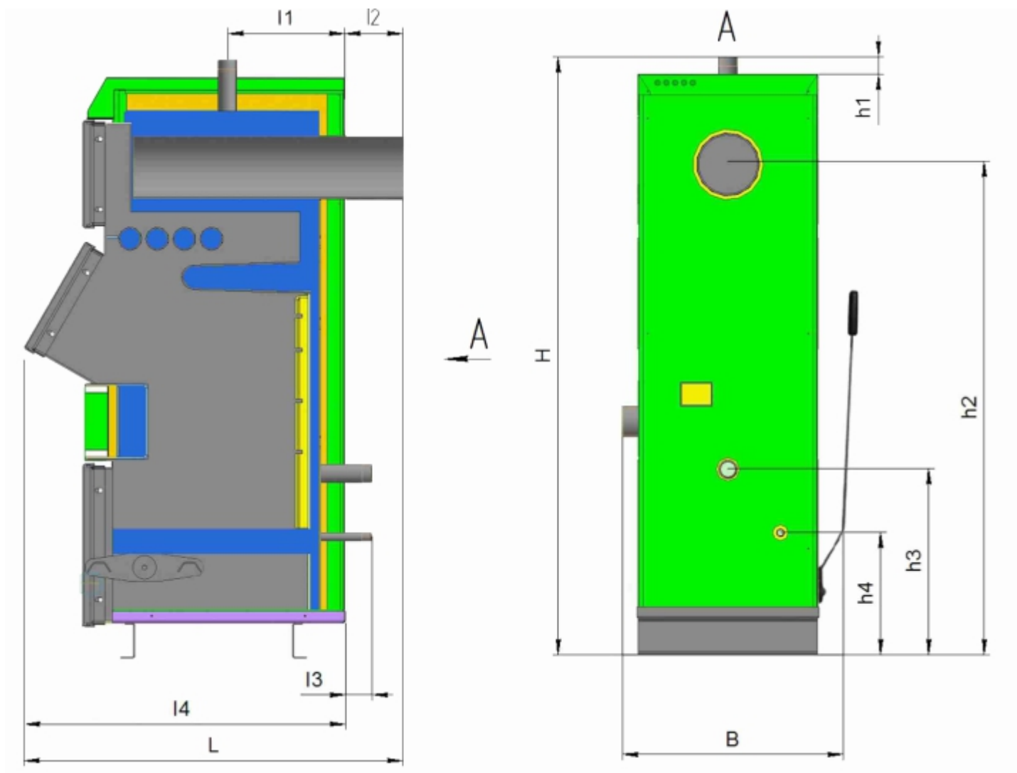
Рисунок 1. Габаритные и присоединительные размеры Котлов моделей LC 12-52
