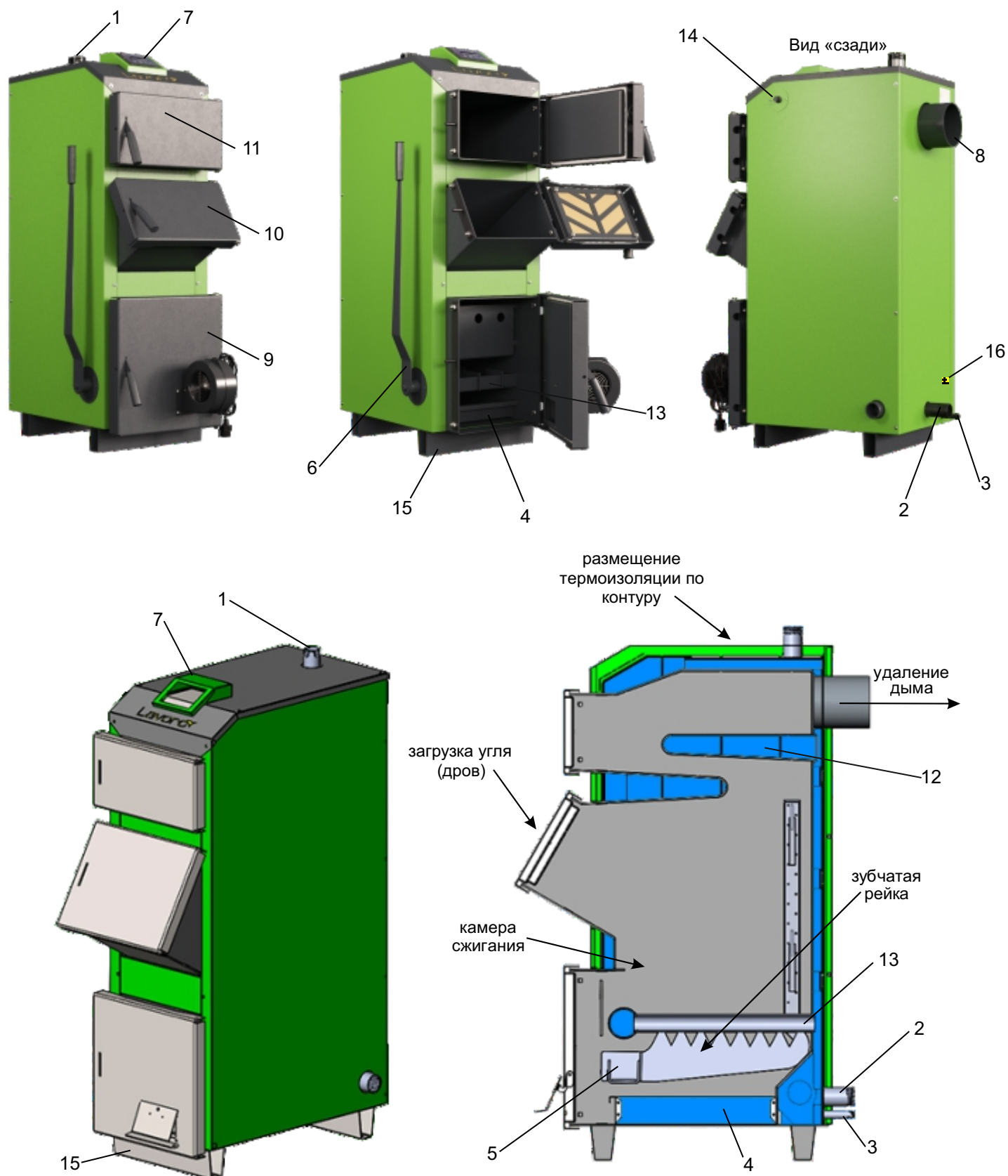
Рисунок 2. Состав и устройство Котлов моделей МС12-32
