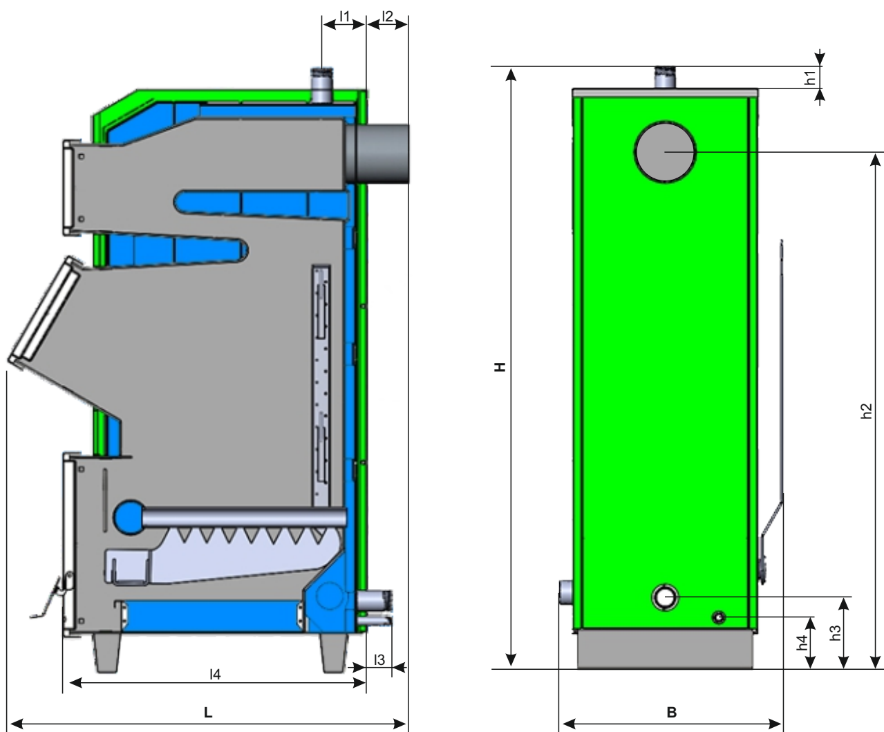
Рисунок 1. Габаритные и присоединительные размеры Котлов моделей MC 12-32
