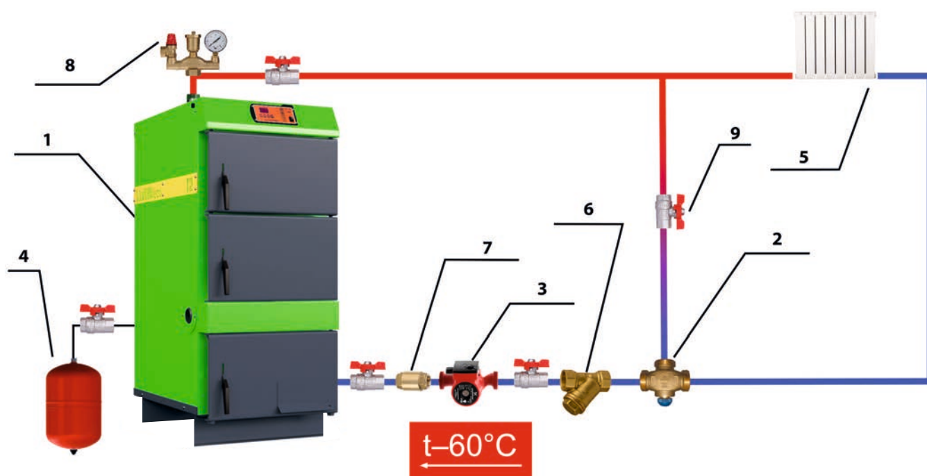
Рисунок 4. Типовая схема обвязки котла Lavoro Eсо с баком-аккумулятором
