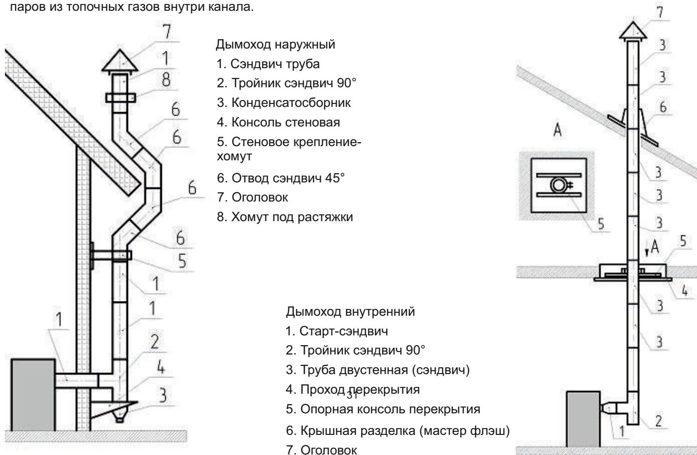
Рисунок Б.1. Пример сборки утепленного (сэндвич) дымохода по конденсату внутри и снаружи помещения
