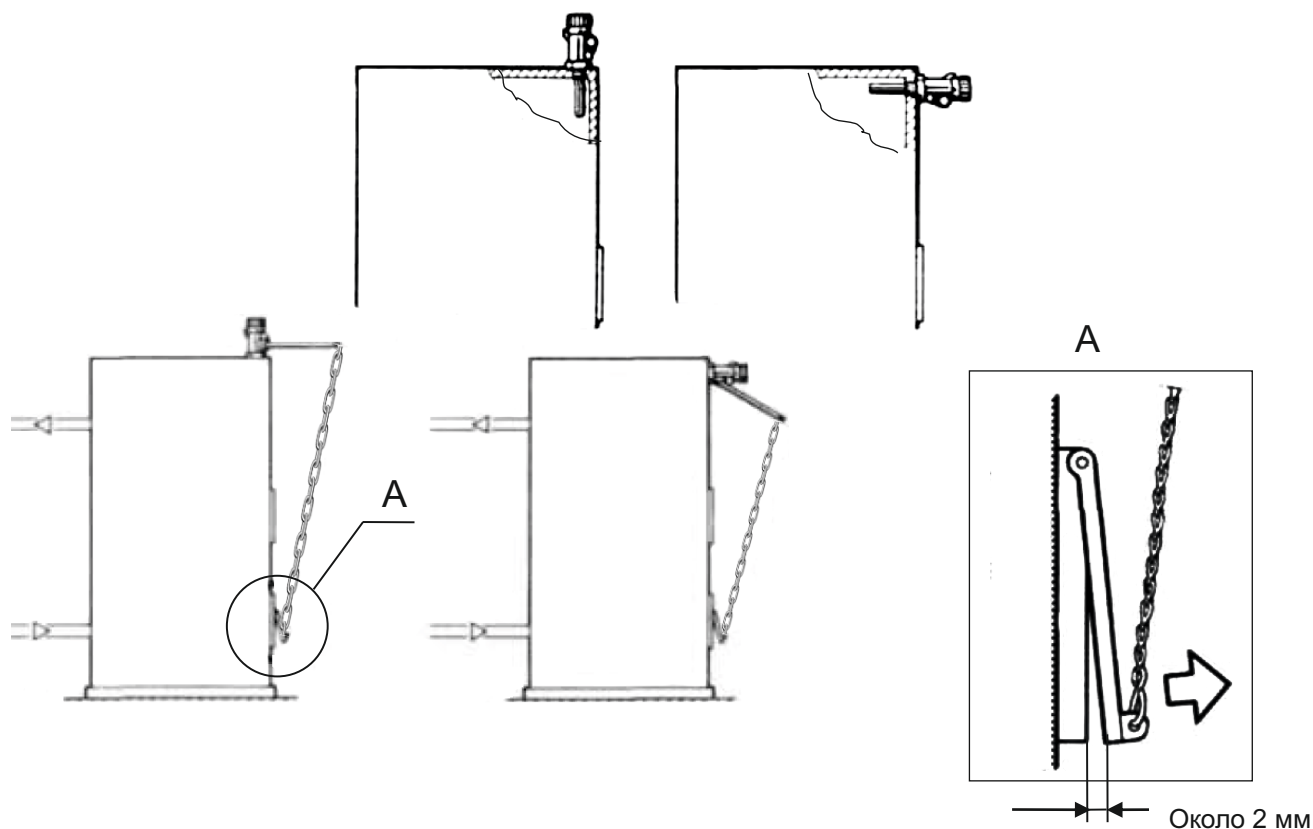
Рисунок 7. Схема закрепления тягорука ятора на заслонке нижней дверцы Котла
