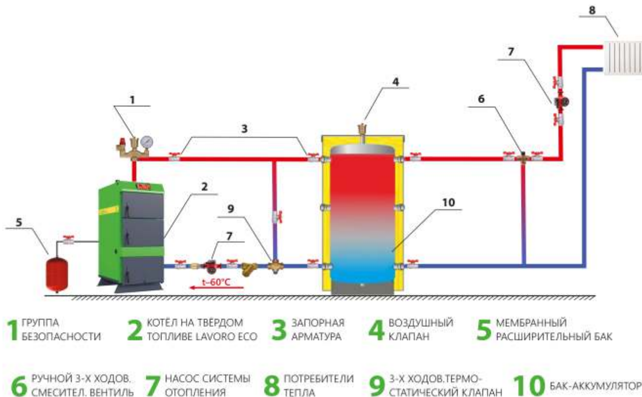
Рисунок 2. Типовая схема обвязки котла Lavoro Eco с баком-аккумулятором
